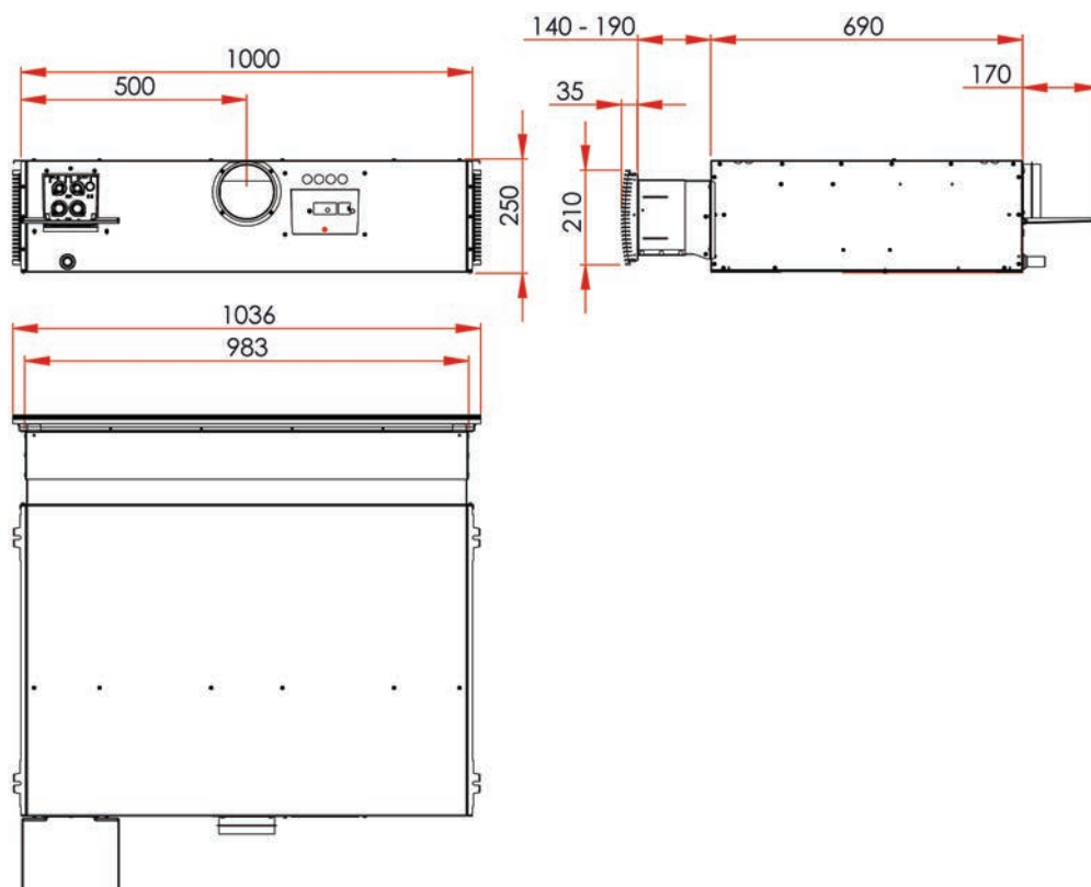
Joonis 4: Grand 100 peamised mõõtmed
