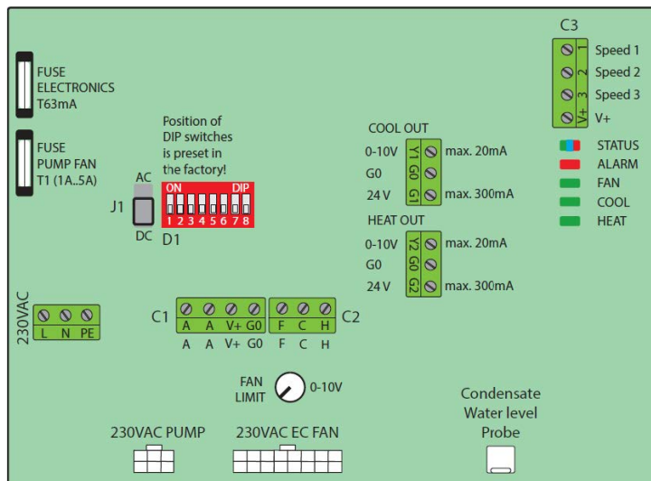
Joonis 6: Vari ühenduspaneel
