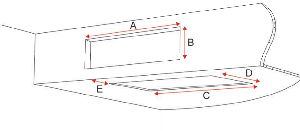
Joonis 13: Paigaldus- ja hooldusluugi avade mõõtmed
