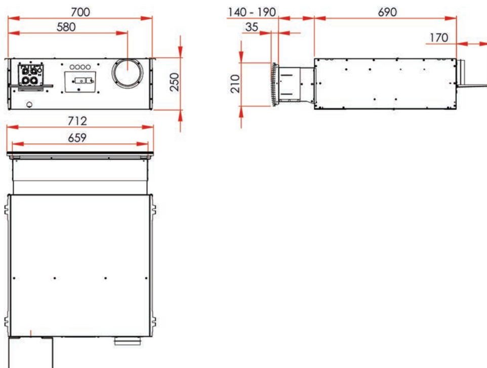
Joonis 3: Grand 70 peamised mõõtmed
