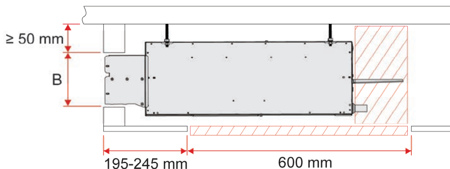
Joonis 12: Paigaldusmõõtmed, küljeltvaade
