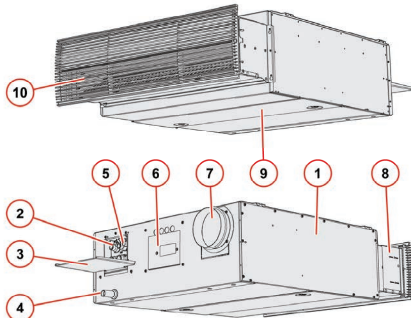
Joonis 1: Seadme ülevaade
