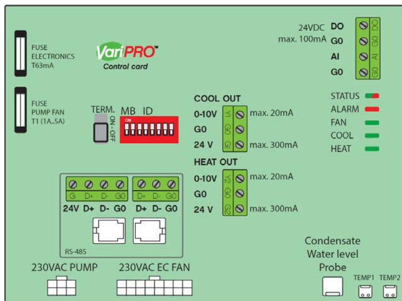
Joonis 8: Vari Pro ühenduspaneel
