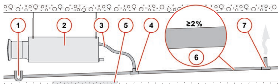
Joonis 14: Kondensveepumba äravoolutorustikuga ühendamise ülevaade
